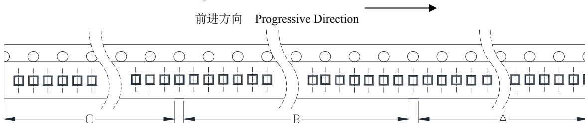
A: 引导, 空带, 300mm; B: 编载产品 20000 只; C: 尾部, 空带, 100mm A: Leader, Empty, 300mm; B: 20000 Lamps Loaded; C: Trailer, Empty, 100mm.
